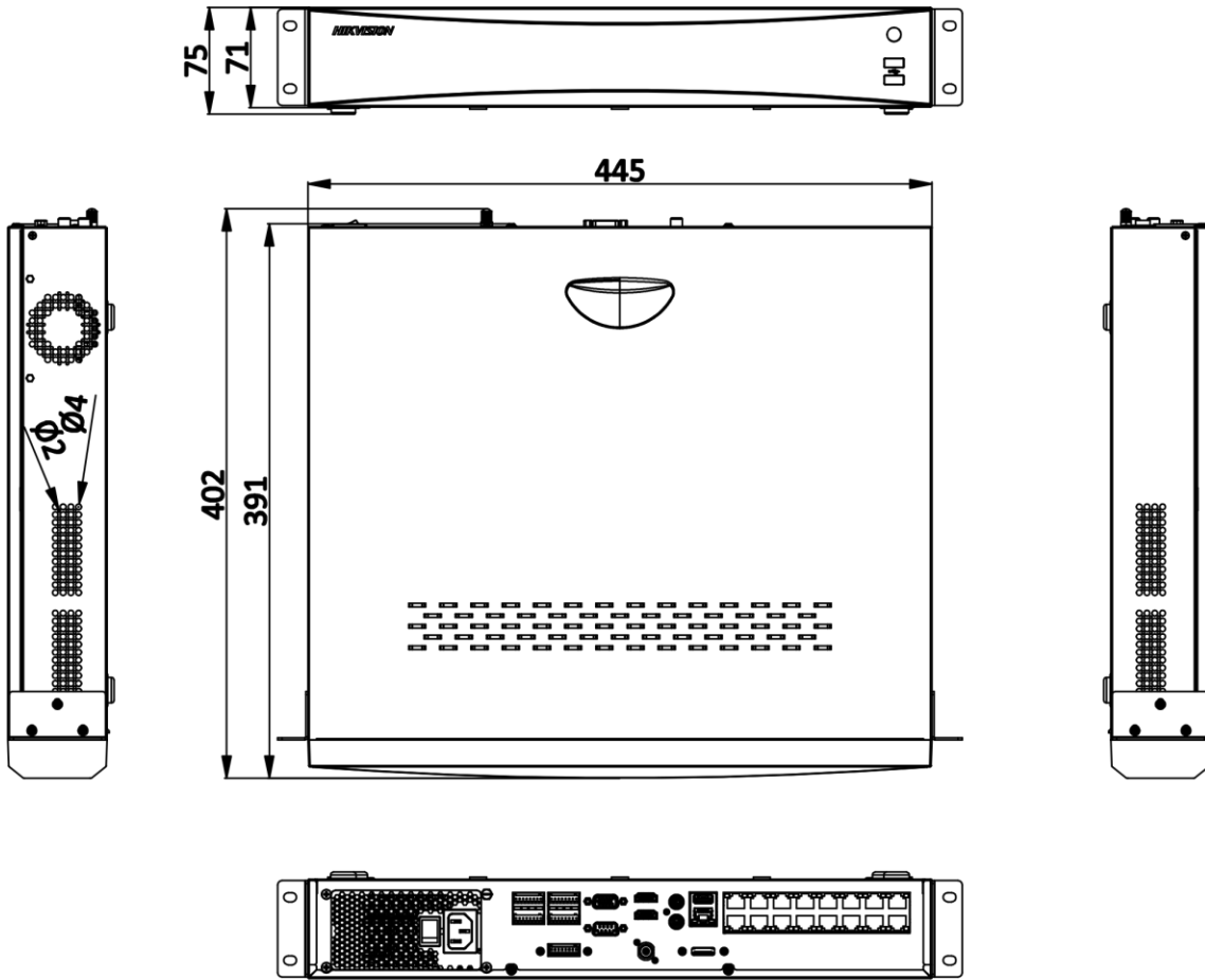
scale/1:1;Unit/mm
